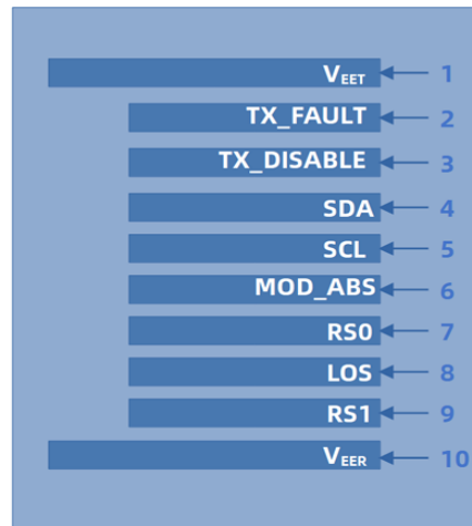
底部直视图
