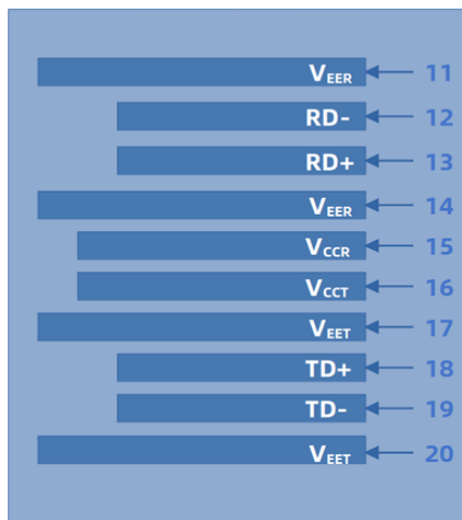
顶部直视图
