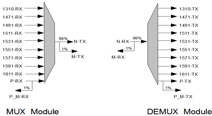
注：上图为 MT2010-CWDM-MUX8-4761-MPG-00 产品的接线图
