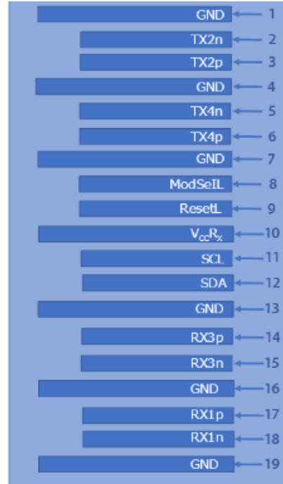
底部直视图
