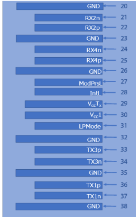
顶部直视图
