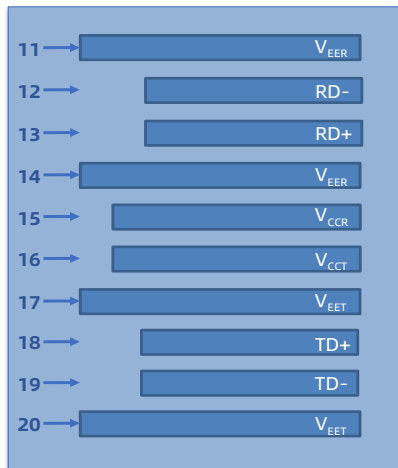
顶部直视图
