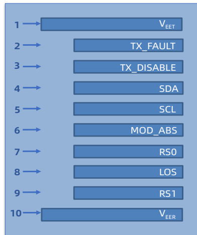
底部直视图
