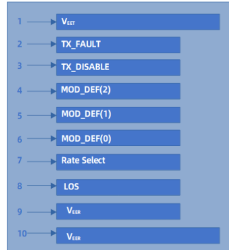
底部视图
